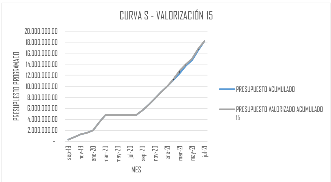
Figura 51: CURVA S - VALORIZACIÓN 15
