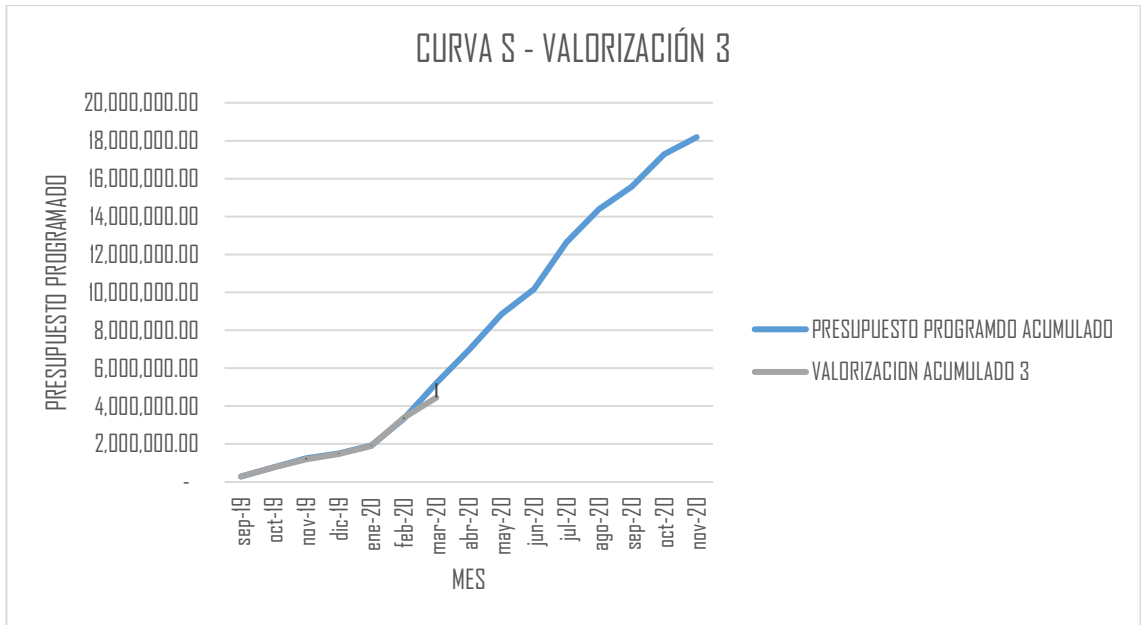
Figura 24: CURVA S - VALORIZACIÓN 3
