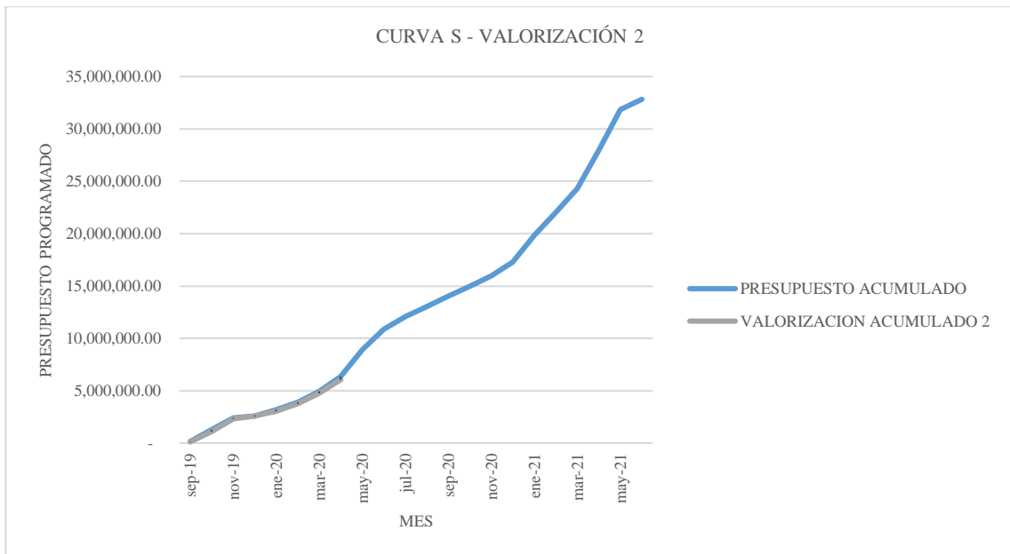
Figura 6: CURVA S - VALORIZACIÓN 2
