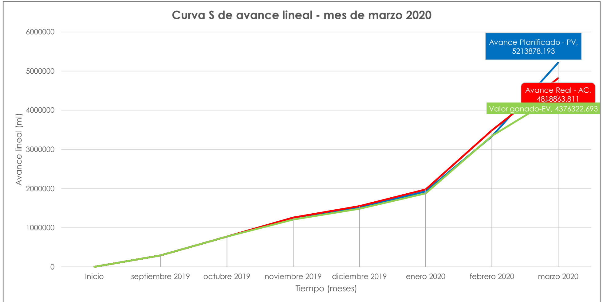
Figura 40: CURVA S - RESUMEN DE AVANCE
