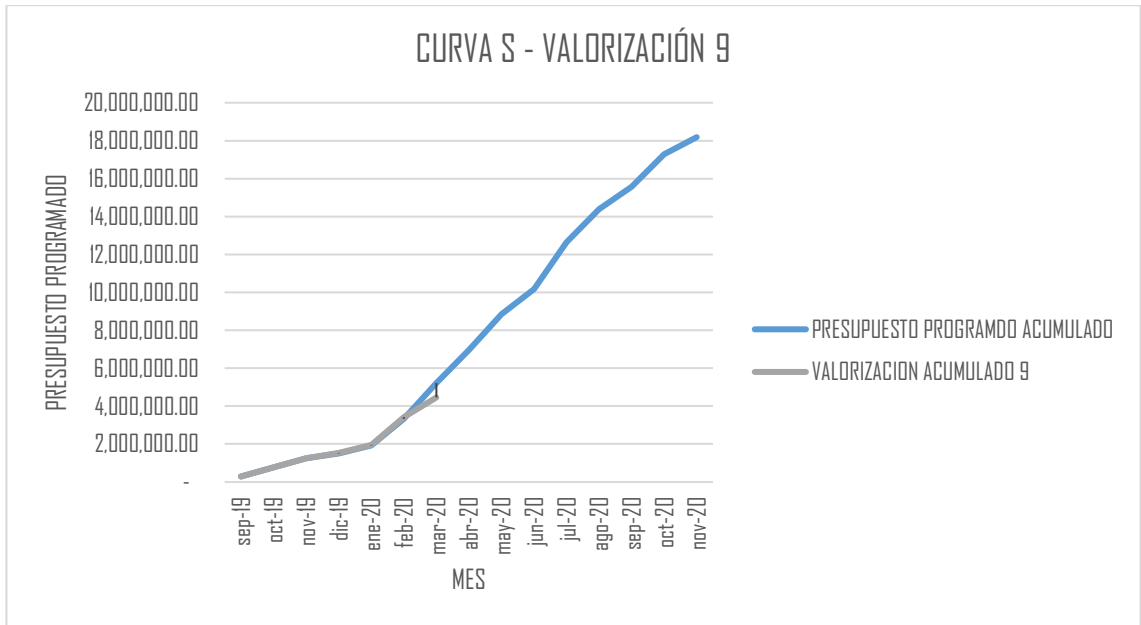
Figura 30: CURVA S - VALORIZACIÓN 9
