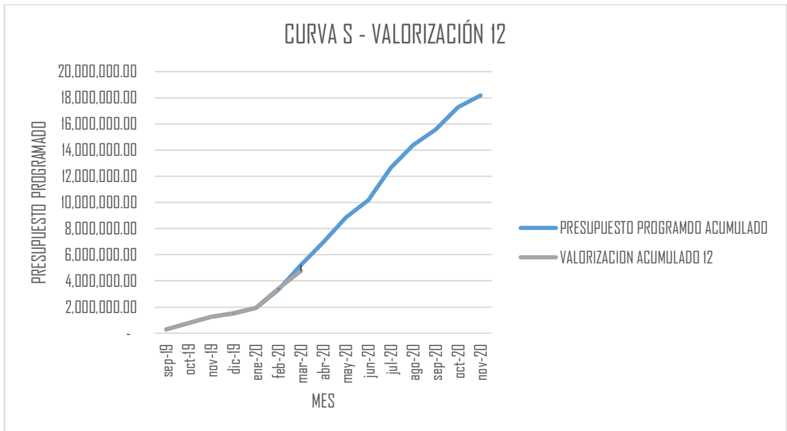
Figura 33: CURVA S - VALORIZACIÓN 12
